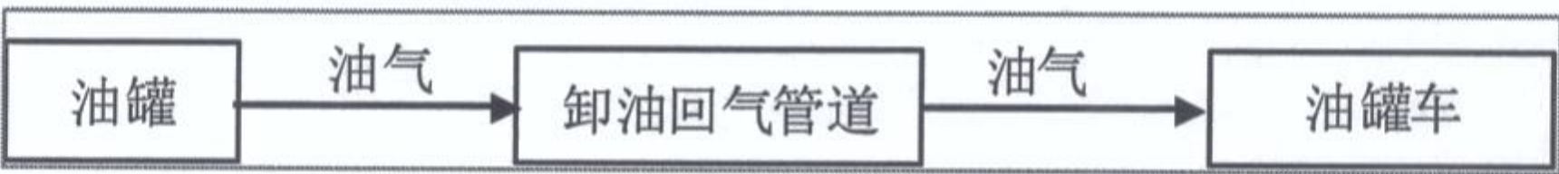
卸油油气回收工艺流程图
