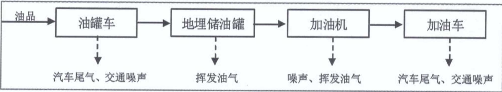
项目运营期工艺流程图
